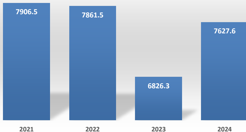
Питоме споживання енергії будівель відділу освіти, кВт*год/м 2
