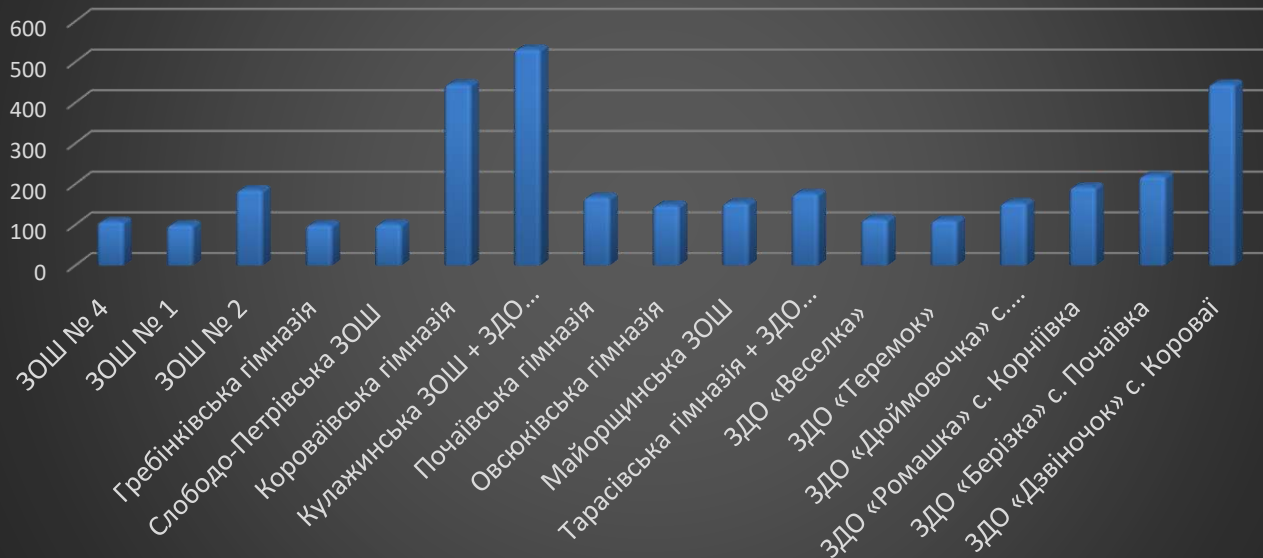
Питоме споживання енергії будівель відділу освіти, кВт*год/м 2
